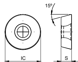
RDHT | RDHW | RDMT | RDMW
