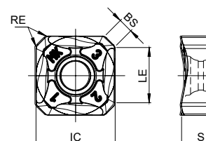
SNH(K)X-MK | LP | MP
