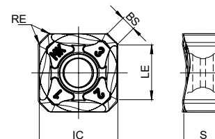
SNH(K)X-MK | MP | LP | LN
